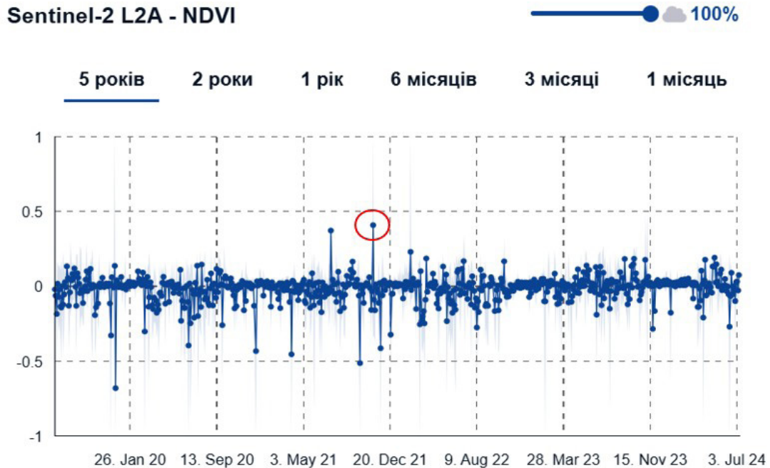
Рис. 6. Гістограма розподілу значень NDVI озера Світязь за період 2020-2024 рр.
