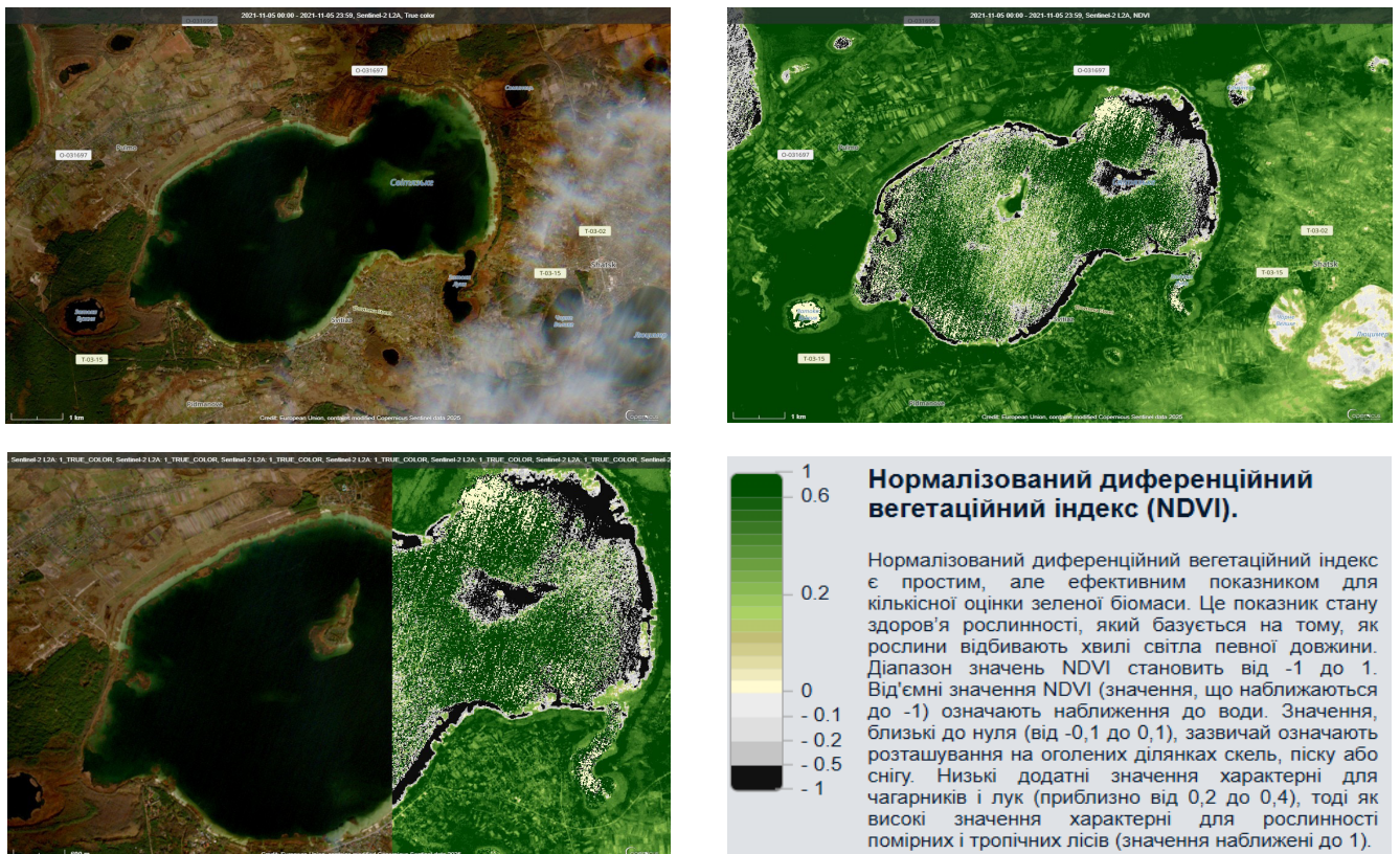
Рис. 7. Значення NDVI озера Світязь станом на 2021.11.05 (космічні знімки Sentinel-2, 2LA)
